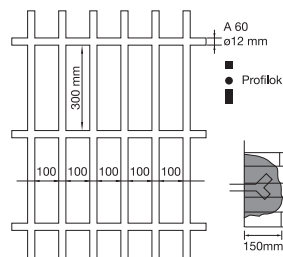
A fixen beépíthető rács kialakításának sémája
