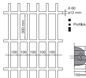
A fixen beépíthető rác kialakításának sémája
